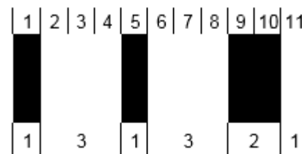
Abbildung 5.4.3.1-2. Symbolzeichenwert 35
