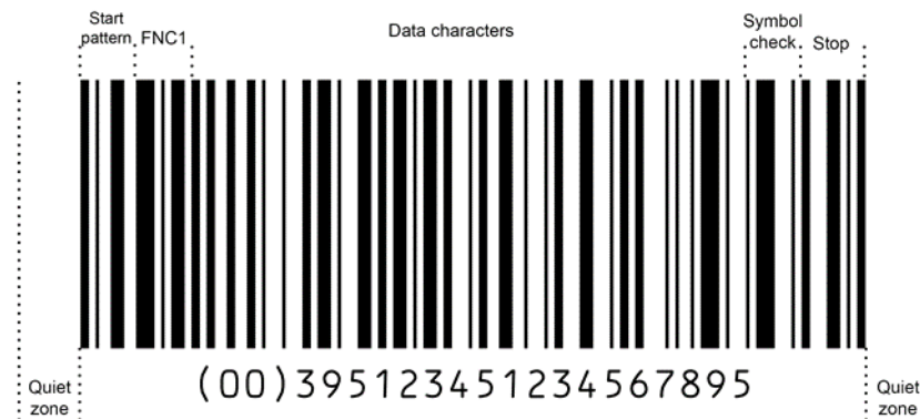
Abbildung 5.4.2-1. Allgemeines Format eines GS1-128 Strichcodes
