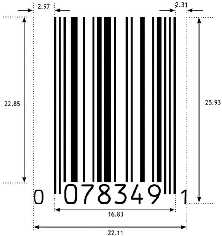
Abbildung 5.2.6.6-4. UPC-E Strichcode
